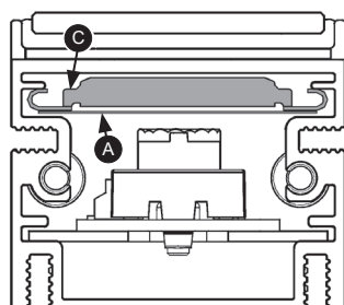
TRASVERSAL LOUVER
