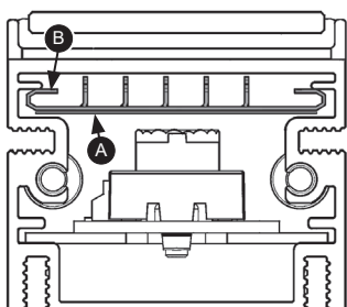
LONGITUDINAL LOUVER
