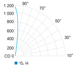
BO WGS (3000K, 80CRI)
