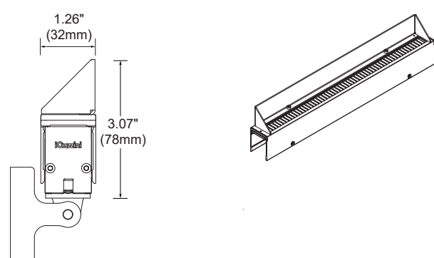
A6- Visor + transversal louver
