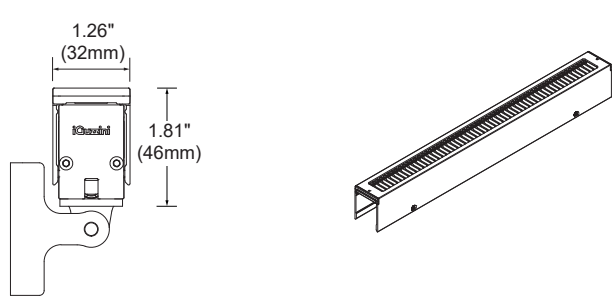
A3- Transversal louver
