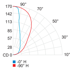
BO WG + no-dot (3000K, 80CRI)
