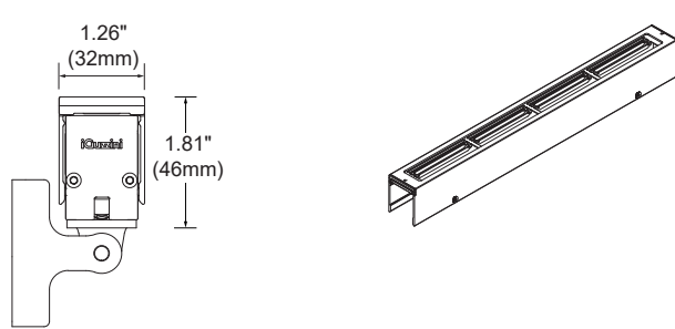
A4- Longitudinal louver
