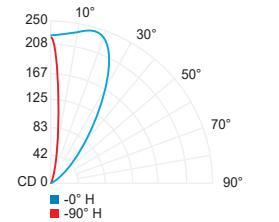
Elliptical 68° / 12° BO (3000K, 80CRI)
